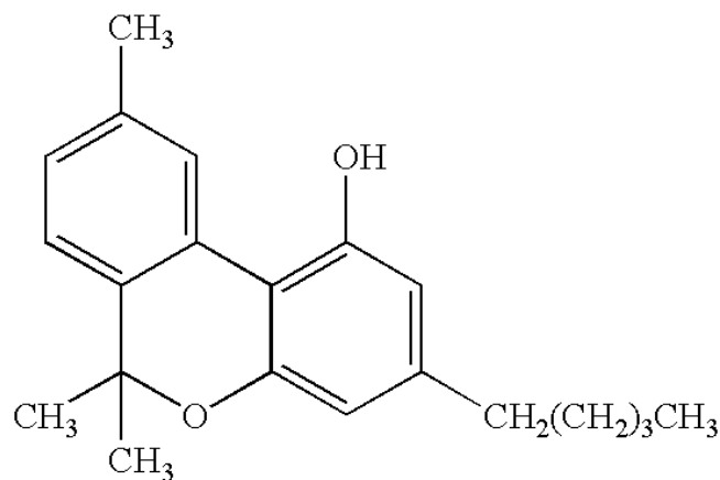
THC
